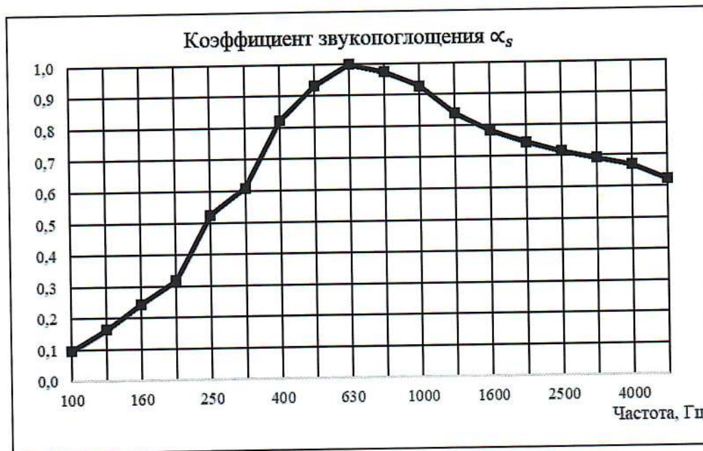
Рис.1 Коэффициент звукопоглощения \alpha_s в третьоктавных полосах частот.
